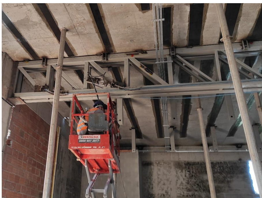
Figura 8 – Foto mostrando macaco aplicando protensão na treliça.
