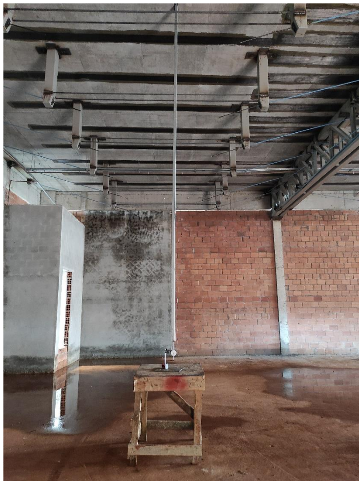
Figura 13 – Foto do defletômetro.
