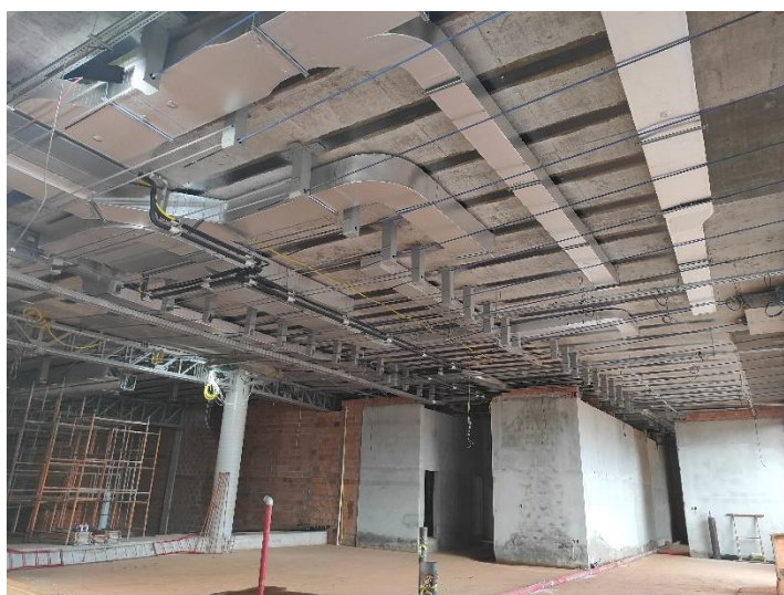
Figura 1 – Foto dos cabos e desviadores para protensão externa da laje
